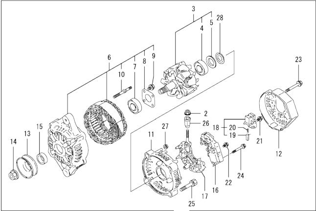
Fig.16. GENERATOR
